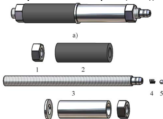
Рисунок Б2 – Схема устройства иньектора а - иньектор в сборе; 1 – гайка; 2 – резиновый уплотнитель (сменный); 3 – трубка иньектора; 4 – пружина; 5 – шарик металлический; 6 – прижимное кольцо (шайба); 7 – прижимная втулка; 8 – прижимная гайка.
